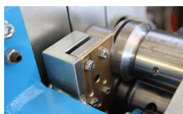
Regolazione materiale dei bordi maschio-femmina
